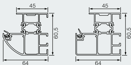
Zarge A1
