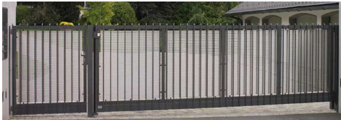
▲ 5 | Schiebetor und Gehtüre mit Edelstahl-Lochblechfüllung und vorgesetzten Zierstäben
